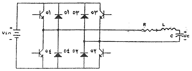
شکل ۹- مدار یک اینورتر ولتاژ
