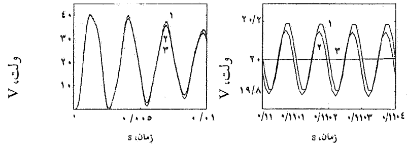
شکل ۸- مبدل چوک (۱: منحنی واقعی، ۲: تقریب مرتبه اول و ۳: روش متوسط گیری فضای حالت) d=0.5
