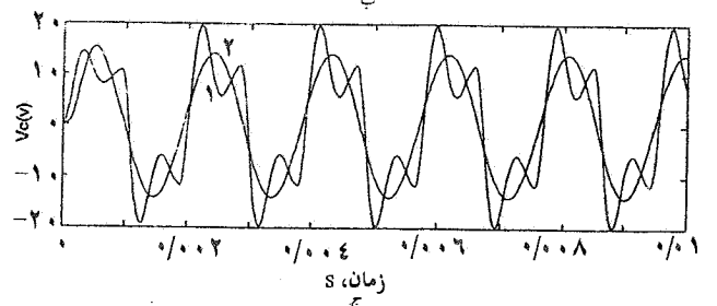
شکل ۱۰- اینورتر موج مربعی (۱): منحنی واقعی و (۲): تقریب با هارمونیک اول
