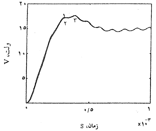
شکل ۲- مبدل کاهنده ولتاژ (۱: منحنی واقعی، ۲: تقریب مرتبه اول و ۳: تقریب مرتبه دوم)
