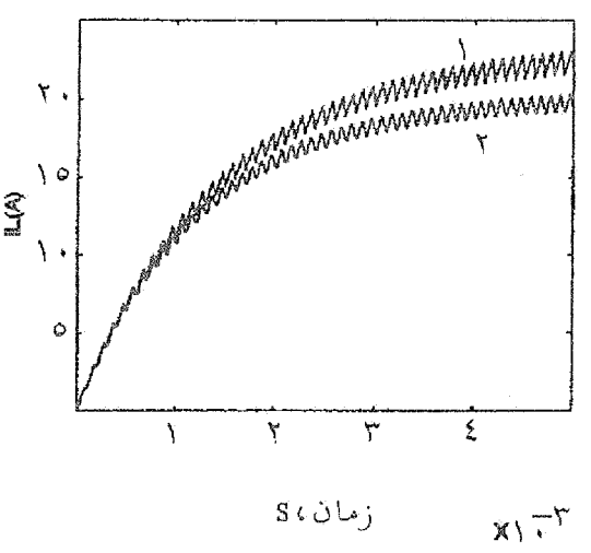
شکل ۶ - مبدل معکوس کننده ولتاژ و ولتاژ (۱) منحنی واقعی و (۲) تقریب مرتبه اول (الف) d=0.25 ، (ب) d=0.5 ، (ج) d=0.75
