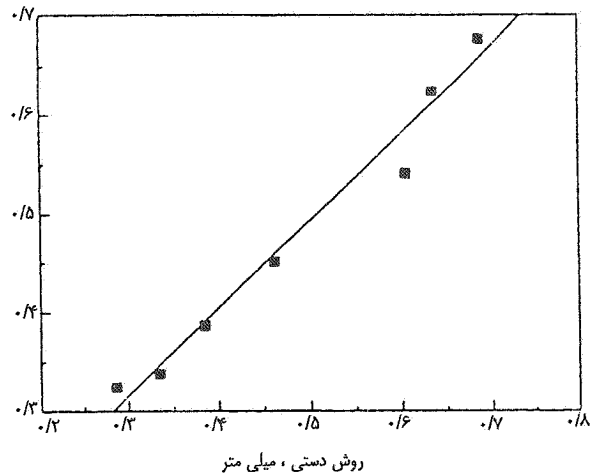
شکل ۱۰ - الف نمودار همبستگی فاصله پودها به روش ACF و دستی
