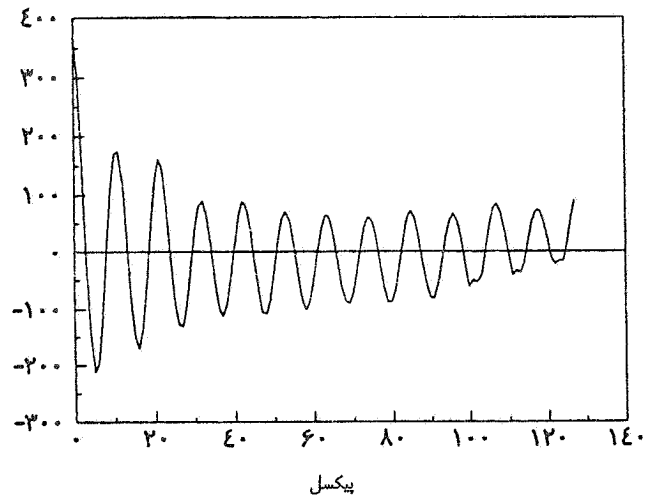
شکل ۸- نمودار خط مرکزی تابع خود همبستگی در جهت
