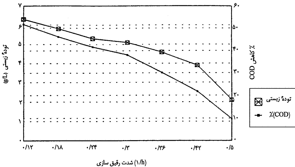
شکل ۸- تغییرات توده زیستی و درصد کاهش XO\Delta با شدت رقیق سازی. دمای 34^{\circ}C ، شدت هوادهی 27.7.m ، دور همزن 0.0. \pi. \mu ، pH اولیه محیط کشت 3/5
