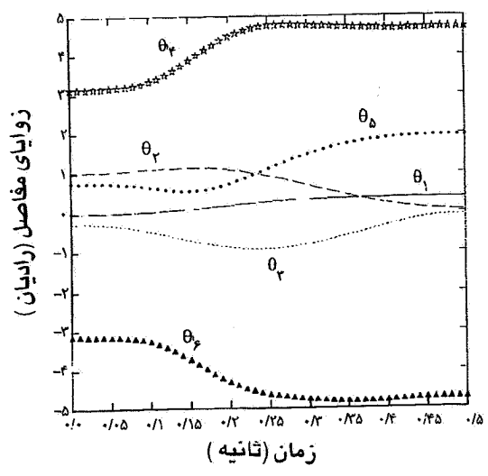
شکل ۳- زوایای مفاصل و نرخ تغییرات آنها برای ربات A
