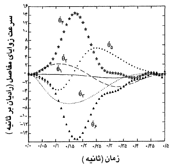
شکل ۴- زوایای مفاصل و نرخ تغییرات آنها برای ربات B
