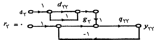
شکل ۲- چهار سیستم SISO معادل با یک سیستم دو متغیره MIMO
