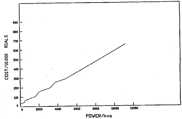
شكل ۳- هزينه پستهای فشار ضعيف برحسب قدرت آنها
