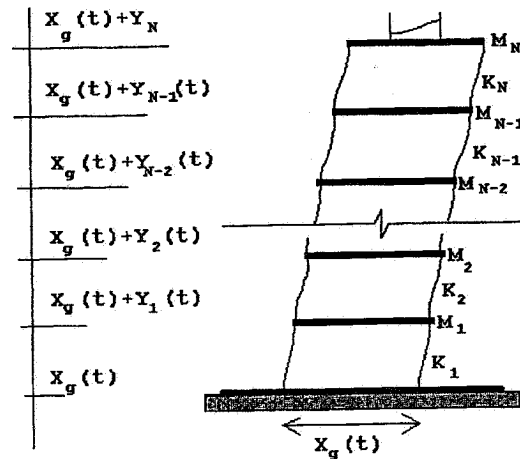
شکل ۲- شبیه‌سازی اندرکنش TLD و سازه N درجه آزادی.
