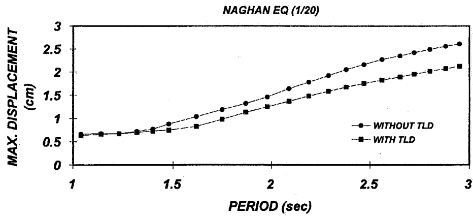
شکل ۱۸- تغییرات پاسخ بیشینه سازه‌ها
