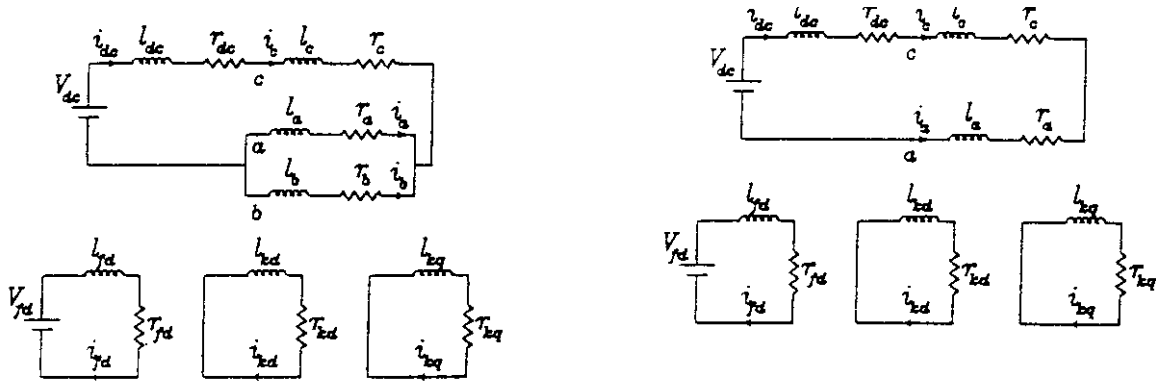
شکل ۳- شمای الکتریکی حالت کاری حین کموتاسیون
