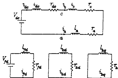
شکل ۲- شمای الکتریکی حالت کاری بین دو کموتاسیون
