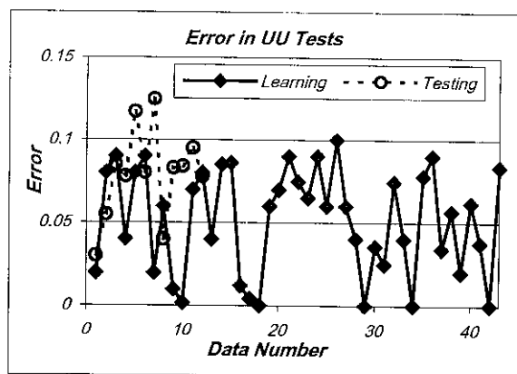
شکل ۵- (الف) روند کاهش خطا با آموزش شبکه در آزمایش UU، (ب) مقایسه خطای داده‌های آزمایشی و آموزشی شبکه
