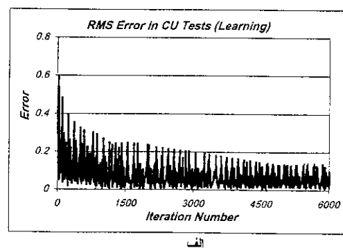
شکل ۹- (الف) روند کاهش خطا با آموزش شبکه در آزمایش CU، (ب) مقایسه خطای داده‌های آزمایشی و آموزشی شبکه
