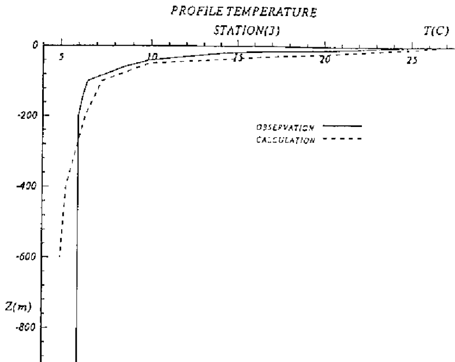
شکل ۸- مقایسهٔ پروفیل دمای حاصل از مشاهده و حل عددی در ایستگاه شماره (۳)
