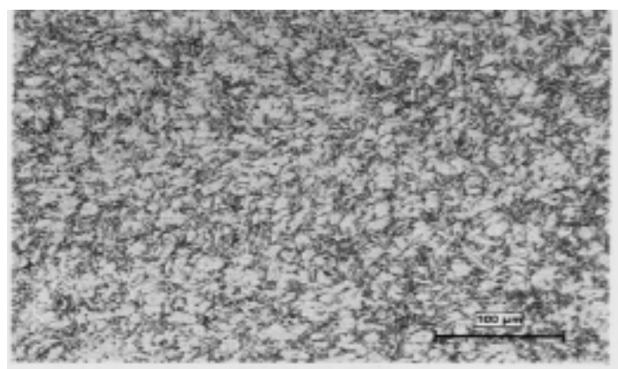
شکل ۱۲- ریز ساختار اولیه نمونه شامل فاز β استحاله یافته ریز در زمینه‌ای از فاز α.
