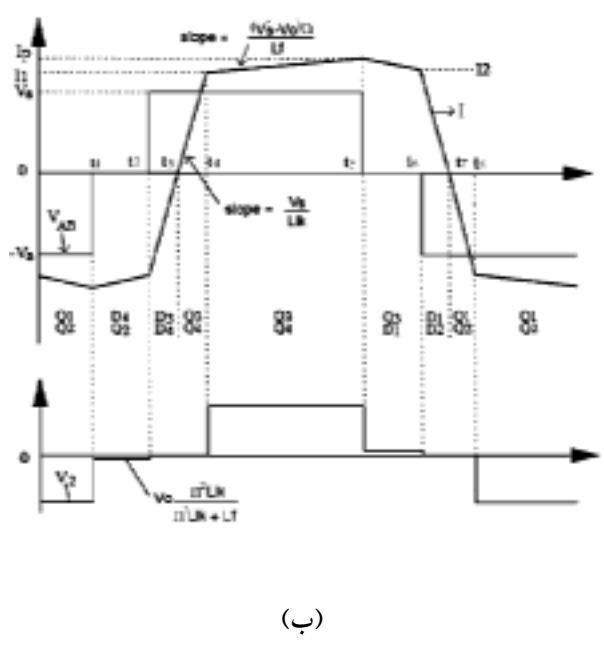
شکل ۱-ب- موجهای آن (روشهای A و B)
