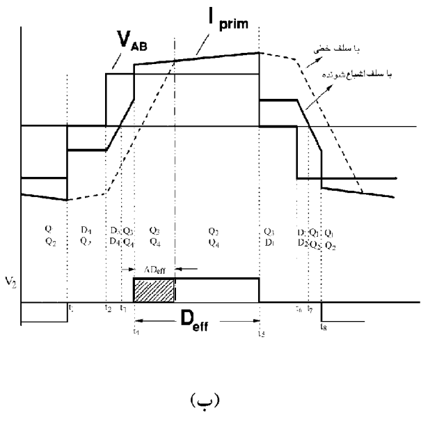
شکل ۲-ب- شکل موجهای آن (روش C)
