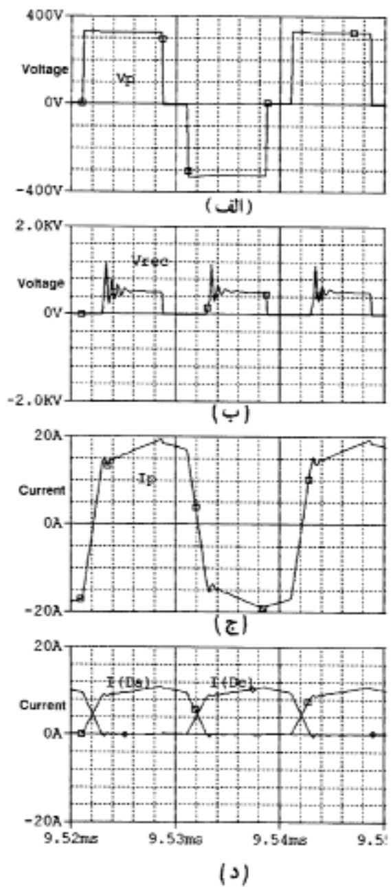
شکل ۶- شکل موجهای مبدل ZVS با سلف نشنی، الف- ولتاژ اولیه ب- ولتاژ ثانویه، ج- جریان اولیه، د- جریان یکسوکننده
