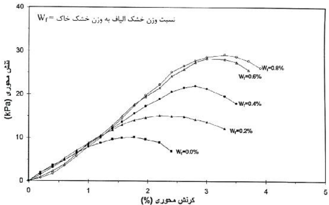
شکل ۱۱- تغییرات تنش بر حسب گرنش محوری در آزمایش تک محوری برای درصدهای وزنی عناصر تسلیح W_f و نسبت اضلاع عناصر A_R=1
