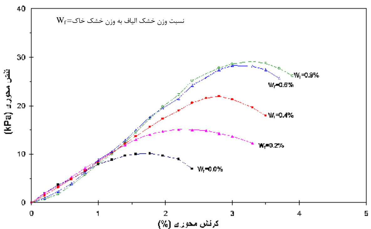
شکل ۱۲- تغییرات تنش بر حسب گرنش محوری در آزمایش تک محوری برای درصدهای وزنی مختلف عناصر تسلیح ( W_f ) و نسبت اضلاع عناصر A_R=3
