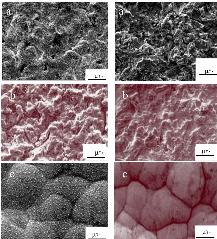
شکل ۱- مورفولوژی سطح نمونه ها، الف- قبل و ب- بعد از عملیات ترموشیمیایی (a) نمونه بدون پوشش (b) نمونه با ۲μ پوشش (c) نمونه با ۴۸nm پوشش
