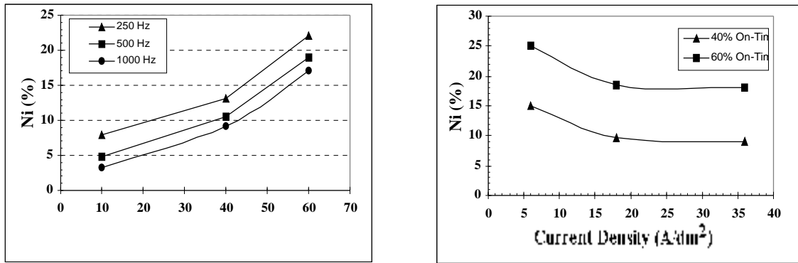
شکل ۵- تغییرات درصد عناصر آلیاژی در پوششهای منقطع بر حسب: راست) چگالی جریان (فرکانس ۵۰۰HZ) (چپ) درصد زمان روشن (بیک چگالی جریان 60 \text{ A/dm}^2 )
