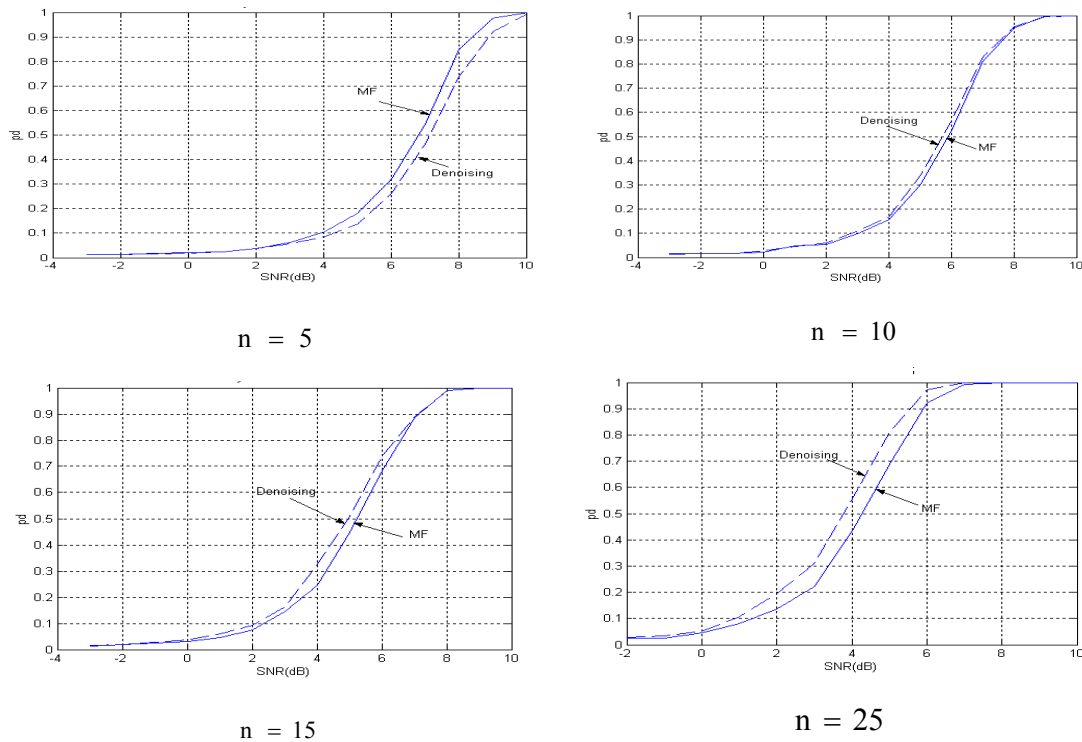
شکل ۸- مقایسه عملکرد فیلتر منطق و نویزدائی در حضور کلاتر غیر سفید برای طول فیلتر ۵ و ۱۰ و ۱۵ و ۲۵
