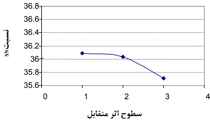
شکل ۱۲- تأثیر اثر متقابل غلظت اسید و دما، ظاهر شده در ستون سوم آرایه بر نسبت SN
