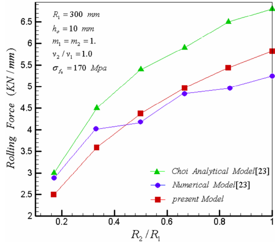
نمودار ۱۵- تغییرات نیروی لازم برای نورد در نسبتهای شعاع مختلف دو غلتک
