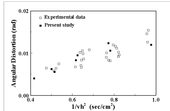
شکل ۱۸- مقایسه نتایج شبیه‌سازیهای انجام شده با داده‌های تجربی جانگ [۵]
