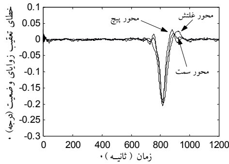
شکل ۱۰- خطای تعقیب زوایای وضعیت
