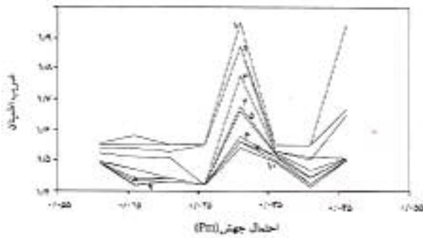
شکل ۹- تغییرات ضرب ضرب اطمینان در برابر احتمال جهش برای ۱۰ بار اجرای برنامه (مثال ۱)
