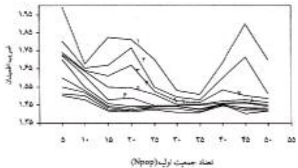
شکل ۱۰- تغییرات ضرب ضرب اطمینان در برابر تعداد جمعیت برای ۱۰ بار اجرای برنامه (مثال ۱)
