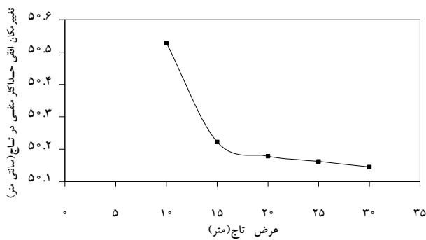
شکل ۳۹- رابطه جابه‌جایی افقی حداکثر منتهی در تاج سد نسبت به عرض تاج سد برای زلزله "ناغان"
