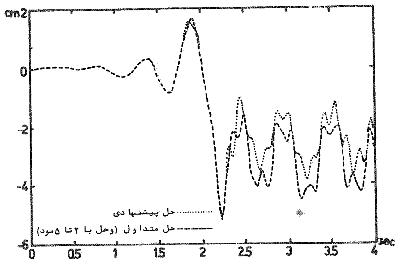
شکل ۷: مقایسه تغییر مکان الاستیک - پلاستیک طبقه با لابه روش حل مستقیم و حل جدید با استفاده از یک مود ارتعاشی با k_b = 40000 و مدول کا رسختی v_y = 1.6 و 1000
