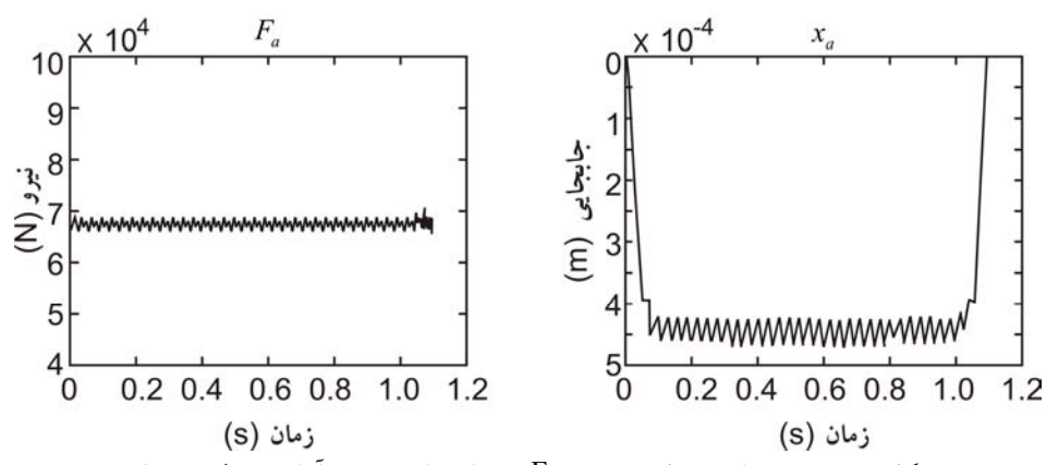
شکل ۶- نیروی تماسی ریل - چرخ F_a و جابه‌جایی درجه آزادی سطح مشترک x_a برای یک تک چرخ عبوری از ریل اصلی
