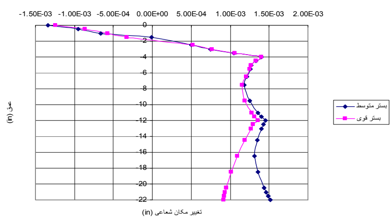
شکل ۴ - مقایسه تغییر مکان شعاعی در دو نوع بستر تحت بار محور ۲۰ تنی، فصل گرم و روسازی نازک
