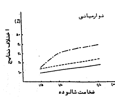
شکل ۸- اثر افزایش ضخامت شالوده بر M_y
