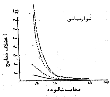
شکل ۹- اثر افزایش ضخامت شالوده بر M_x
