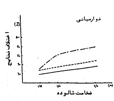
شکل ۸- اثر افزایش ضخامت شالوده بر M_y
