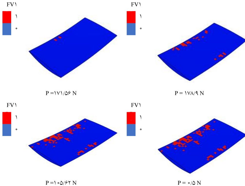
شکل ۷- نحوه رشد FV1 برای پود تحت بارگذاری کششی
