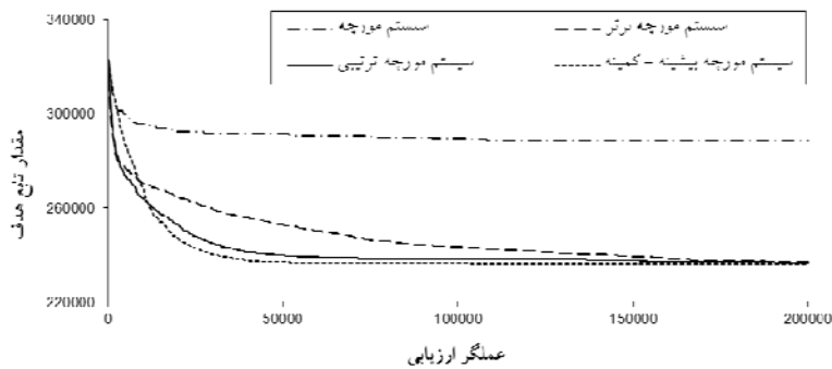
شکل ۷- تغییرات میانگین مقدار تابع هدف مسأله نمونه اول (I) با استفاده از فرمول‌بندی دوم الگوریتم‌های مختلف پیشنهادی
