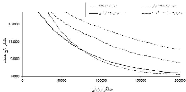
شکل ۸- تغییرات میانگین مقدار تابع هدف مسأله نمونه دوم (II) با استفاده از فرمول‌بندی دوم الگوریتم‌های مختلف پیشنهادی
