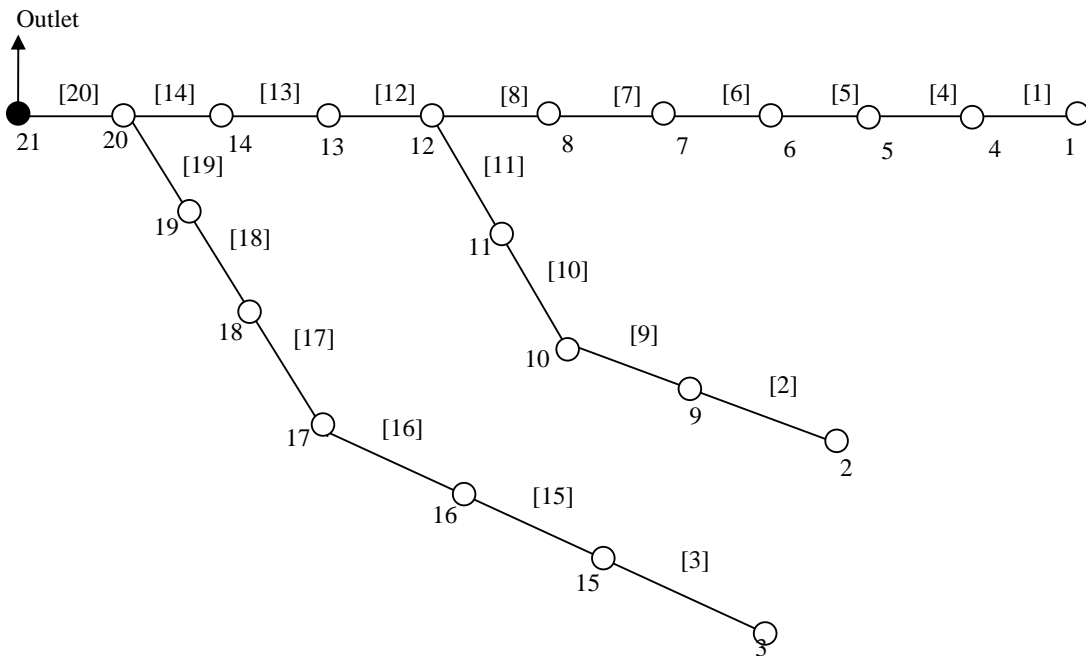
شکل ۴- جانمایی شبکه مسأله نمونه دوم (II)
