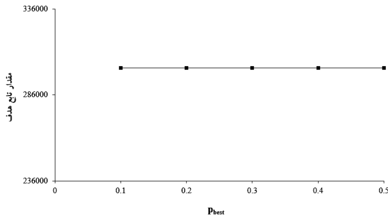
شکل ۱۱- میانگین مقدار تابع هدف مسأله نمونه اول (I) با استفاده از فرمول‌بندی اول الگوریتم سیستم مورچه‌بیشینه- کمینه‌به‌زای Pbest مختلف
