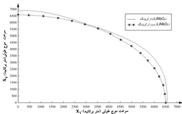
شکل ۷- سرعت فاز در ماده پیزوالکتریک لیتیوم نیوباته الاستیک برای موج طولی در صفحه X_3 = 0 با در نظر گرفتن کوپلینگ پیزوالاستیک (خط ستاره‌دار) و در حالت فقط الاستیک (خط ممتد)
