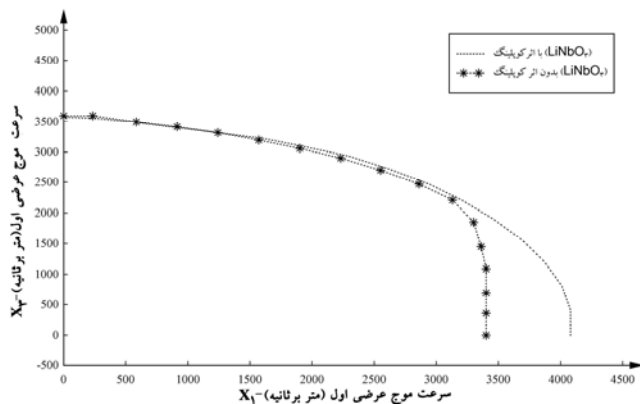
شکل ۵- سرعت فاز در ماده پیزوالکتریک لیتیوم نیوباته الاستیک برای موج عرضی عمودی (اول) در صفحه X_3 = 0 با در نظر گرفتن کوپلینگ پیزوالاستیک (خط چین) و در حالت فقط الاستیک (خط چین ستاره‌ای)
