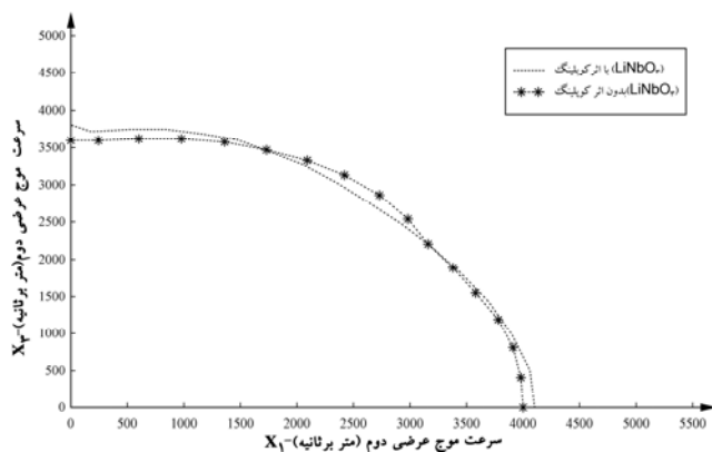
شکل ۶- سرعت فاز در ماده پیزوالکتریک لیتیوم نیوباته الاستیک برای موج عرضی دوم (افقی) در صفحه X_3 = 0 با در نظر گرفتن کوپلینگ پیزوالاستیک (خط چین) و در حالت فقط الاستیک (خط چین ستاره‌ای)
