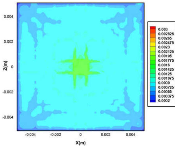
شکل ۶- توزیع کسر حجمی نانوذرات اکسید مس در انتهای کانال ( y = 50 \text{ cm} ) در کسر حجمی متوسط \phi = 0/1\% و
