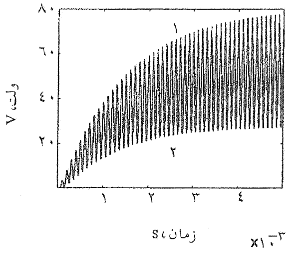
شکل ۶- مبدل معکوس کننده ولتاژ و لنتاز (۱: منحنی واقعی و ۲: تقریب مرتبه اول) (الف) d=0.25 ، (ب) d=0.5 و (ج) d=0.75
