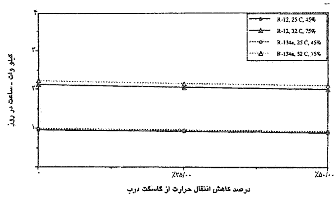
شکل ۸- تاثیر کاهش انتقال گرما از واشر دور درب روی مصرف برق یخچال نمونه
