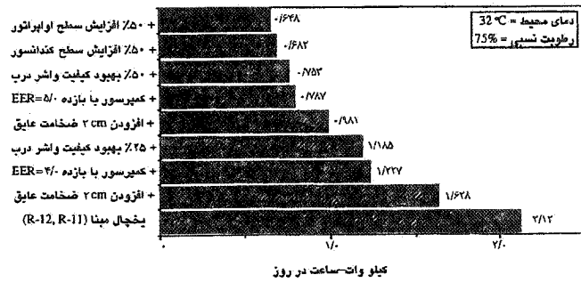
شکل ۱۱- تاثیر اجرای طرحهای انتخابی روی مصرف برق یخچال نمونه (دمای محیط 32°C، رطوبت نسبی 75%)
