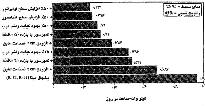
شکل ۱۰- تاثیر اجرای طرحهای انتخابی روی مصرف برق یخچال نمونه (دمای محیط 25°C، رطوبت نسبی 45%)
