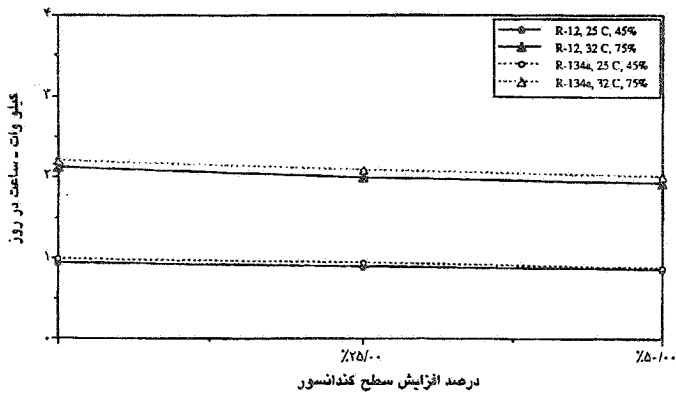
شکل ۷- تاثیر افزایش سطح گرمایی کندانسور روی مصرف برق یخچال نمونه
