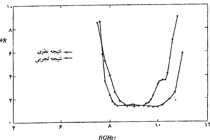
شکل ۷- نتیجه تجربی و نظری برای VSWR آنتن مثال (۴)، w_a=0/4\text{cm} ، d_a=0/75\text{cm} ، b=1/1\text{cm} ، a=0/7\text{cm} ، d_1=0/31\text{cm} ، \epsilon_{rf}=6/15 ، w_f=0/9\text{cm} ، d_s=0/11\text{cm} ، d_f=0/614\text{cm}
