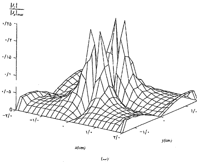
شکل ۵- توزیع جریان روی آنتن، l_a=1/1 , b=3\text{cm} , a=4\text{cm} , x_p=y_p=0 , l_s=1/2\text{cm} , w_f=0.44\text{cm} , w_a=0.16\text{cm} مستقارن، f=2/23\text{GHz} و d_1=d_f=0.16\text{cm} , \epsilon_{rf}=\epsilon_{rf}=2/54 (الف) - مؤلفه x (ب) - مؤلفه y
