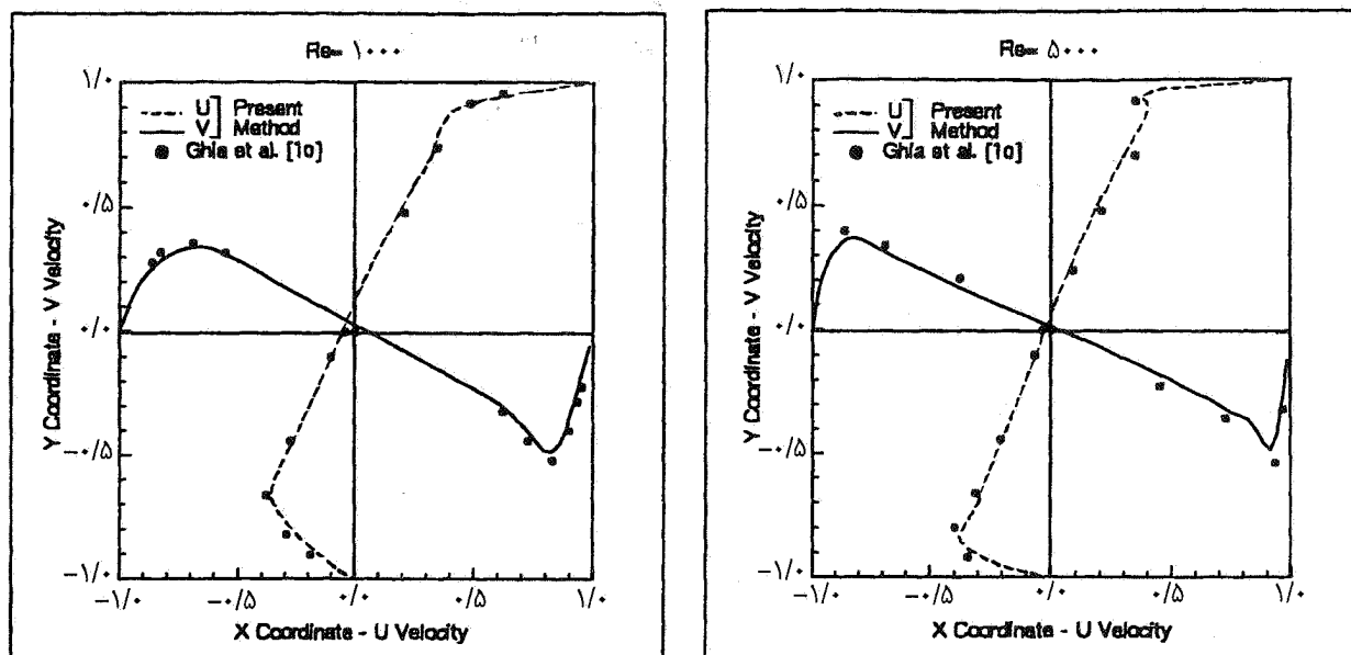
شکل ۱- مقایسه نتایج مسئله حفره و کار عددی مشابه [۱۰]
