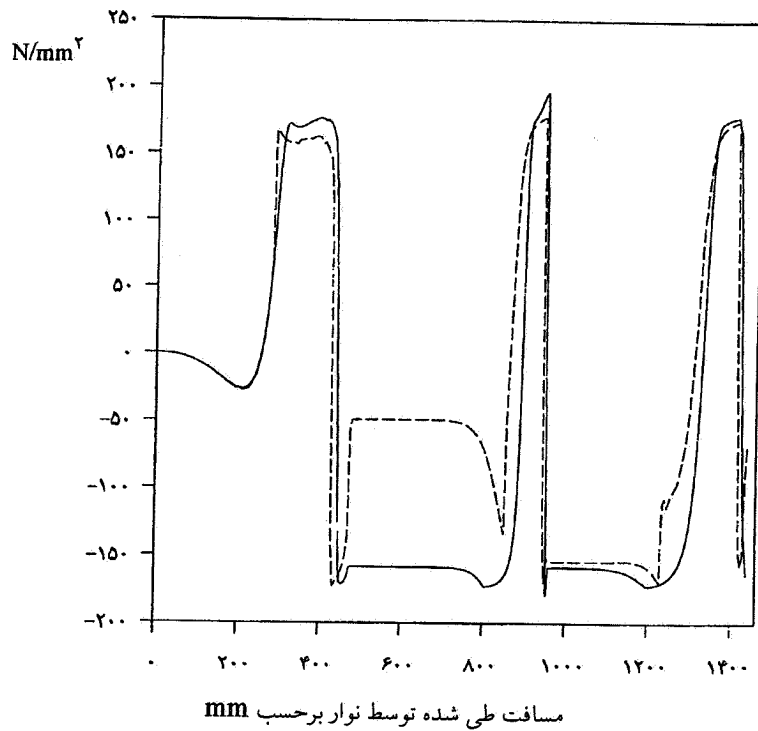
شکل ۶- نتایج تحلیلی تنش طولی نقطه‌ای واقع بر لایه بالایی و لبه بال مقطع مربوط به نمونه آزمایشهای فیوترل نتایج با استفاده از معادله‌های لوی - میسز به تنهایی ----- نتایج با استفاده از معادله‌های پراندل روس —————
