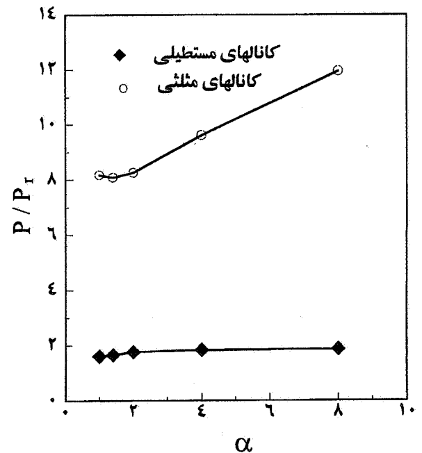
شکل ۱۱- تغییرات نسبت توان پمپاژ کانالهای مستطیلی و مثلثی به توان پمپاژ کانالهای سطح مینا بر حسب \alpha در حالت VG-۳
