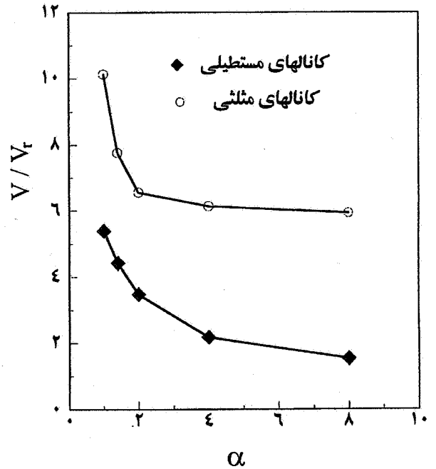
شکل ۹- تغییرات نسبت حجم مبدل برای کانالهای مستطیلی و مثلثی به حجم مبدل سطح مینا بر حسب \alpha در حالت VG-۱
