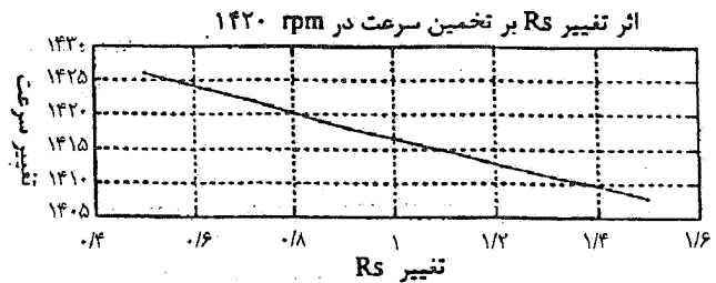
شکل ۶- اثر تغییر R_s بر روی تخمینگر سرعت در 1420 \text{ rpm}
