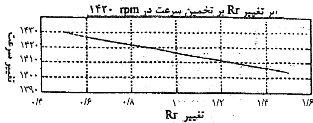
شکل ۷- اثر تغییر R_r بر روی تخمینگر سرعت در 1420 \text{ rpm}
