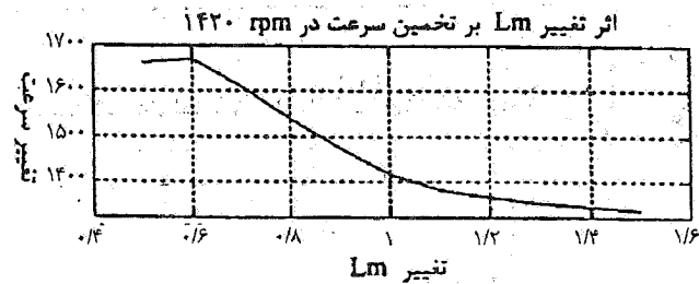
شکل ۸- اثر تغییر L_m بر روی تخمینگر سرعت در 1420 \text{ rpm}
