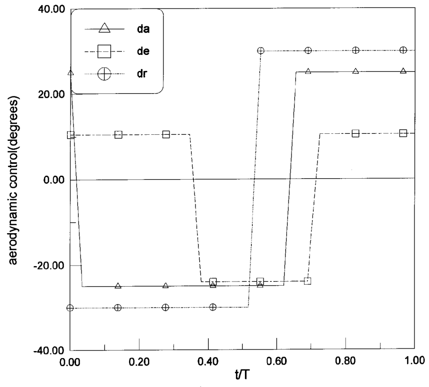
شکل ۵- کنترل‌های آیرودینامیکی
