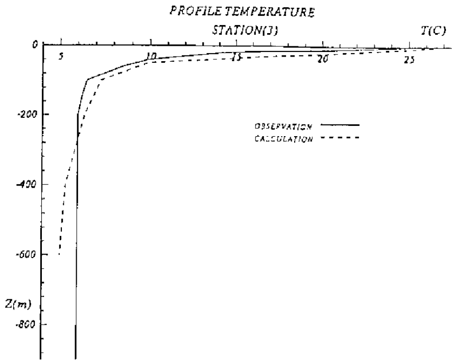
شکل ۸- مقایسهٔ پروفیل دمایی حاصل از مشاهده و حل عددی در ایستگاه شماره (۳)
