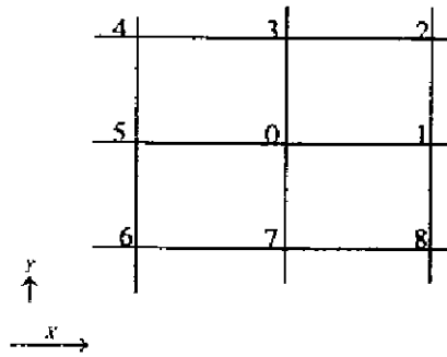
شکل ۱- نمایش شماتیک شبکه و وضعیت گره ها برای استفاده در روش تفاضلهای محدود توجه: S = فاصله بین گره ها است.
