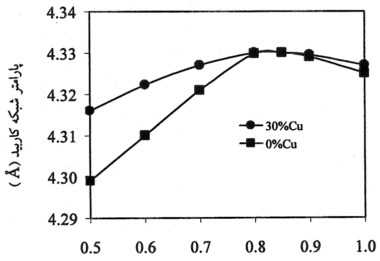
شکل ۳- پارامتر شبکه کاربید تیتانیوم بر حسب تابعی از نسبت C/Ti در مخلوط اولیه، با و بدون حضور مس
