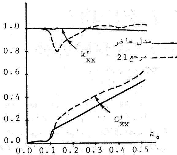
شکل ۳- سختی دینامیکی افقی شمع منفرد
