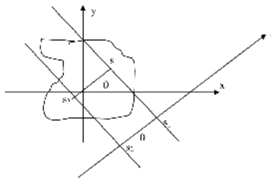
شکل ۱- چگونگی محاسبه تبدیل رادن از یک تصویر دوبعدی آنالوگ
