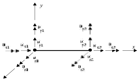
شکل ۵- عنصر قاب و درجات آزادی گره‌ای آن در حالت سه بعدی
