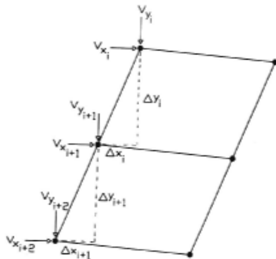
شکل 4- محاسبه دبی تراوش از دو جزء قرار گرفته در بالادست
