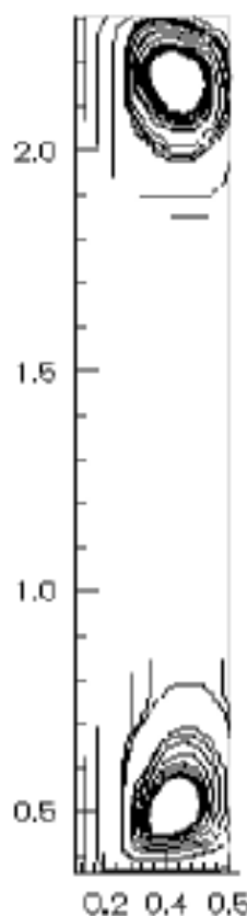
شکل ۳- جریان ثانویه در مقطع کانال در ناحیه توسعه یافته
