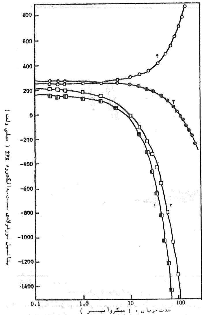
شکل ۴ تغییر پتانسیل تور فولادی بعنوان تابعی از شدت جریان برای پلاریزاسیون کاتدی صفحه فولادی . منحنی‌های ۴۰۳،۲۰۱ بر ترتیب پتانسیل تور فولادی در موقعیت ۴۰۳،۲۰۱ نسبت به الکترو د 2PX در موقعیت ۴ را نشان میدهد .
