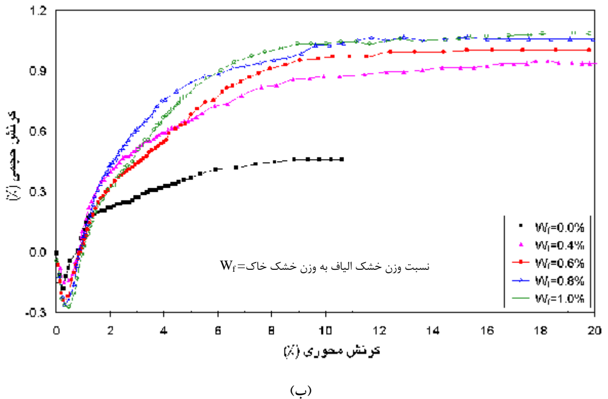
شکل ۵- تغییرات تنش انحرافی (شکل الف) و کرنش حجمی (شکل ب) در آزمایش سه محوری CD ( s'_c = 100 \text{ kPa} ) برای درصدهای
