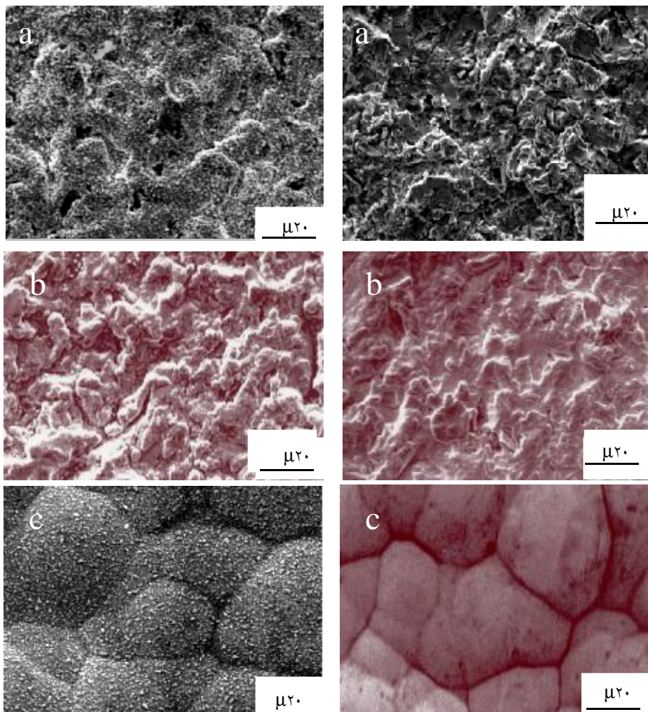
شکل ۱- مورفولوژی سطح نمونه ها، الف- قبل و ب- بعد از عملیات ترموشیمیایی (a) نمونه بدون پوشش (b) نمونه با ۲μm پوشش (c) نمونه با ۴μm پوشش
