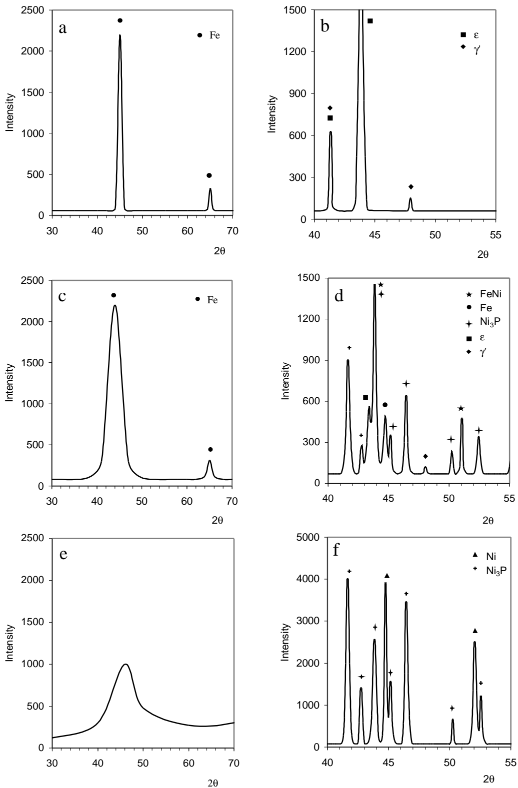
شکل ۳- نتایج تفرق اشعه ایکس نمونه‌ها، قبل و پس از فرایند ترموشیمیایی بدون پوشش، (a,b) با ۲ میکرون پوشش، (c,d) با ۴ میکرون پوشش، (e,f) با ۸ میکرون پوشش
