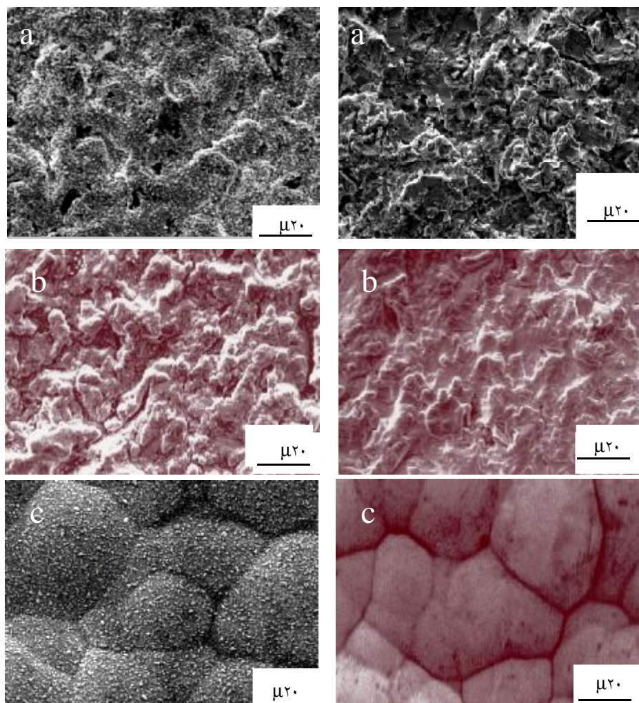
شکل ۱- مورفولوژی سطح نمونه ها، الف- قبل و ب- بعد از عملیات ترموشیمیایی (a) نمونه بدون پوشش (b) نمونه با ۲μ پوشش (c) نمونه با ۸μ پوشش
